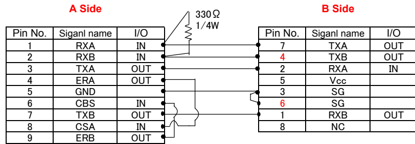
图: 結線图
